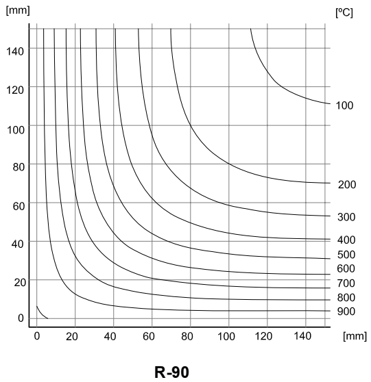
Figura C.6. Isothermas para cuartos de sección de 300 x 300 mm expuestos por ambas caras
