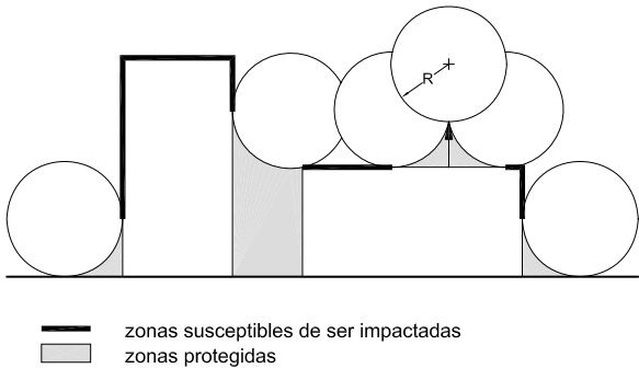
Figura B.3 Esfera rodante en estructuras
